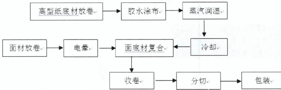
图 3.3 生产工艺流程图
