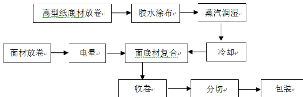
图 3.3 生产工艺流程图
